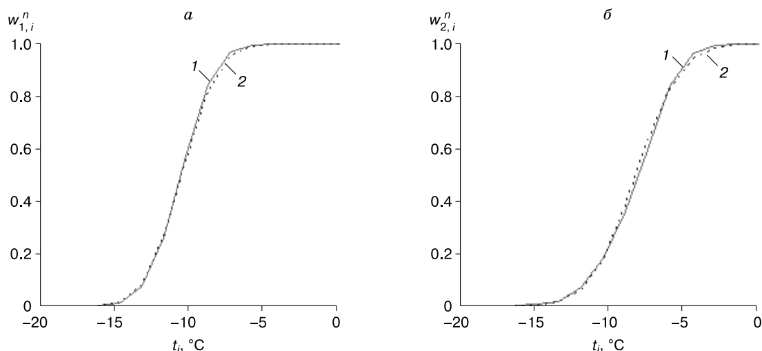
Рис. 2. Сравнение эмпирических (1) и нормальных (2) распределений вероятности найти температуру меньше заданной ( t ):
