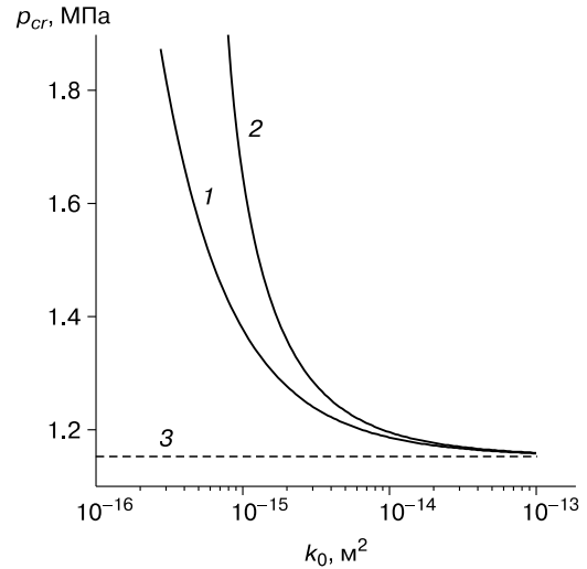
Рис. 6. Зависимость предельного значения давления нагнетаемого газа p_{cr} от абсолютной проницаемости пласта k_0 .
