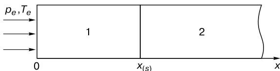
Рис. 1. Схема процесса инъекции диоксида углерода.
