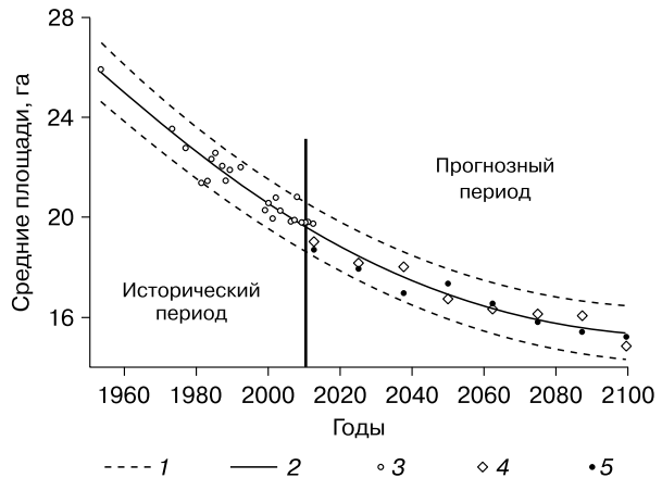
Рис. 9. Прогнозирование динамики среднего значения площади термокарстовых озер в зоне многолетней мерзлоты Западной Сибири.
