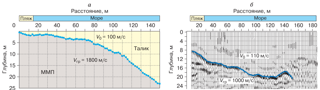
Рис. 2. Примеры использования преломленных (а) и отраженных (б) поперечных SH -волн для изучения таликов в пределах мелководной части шельфа.
