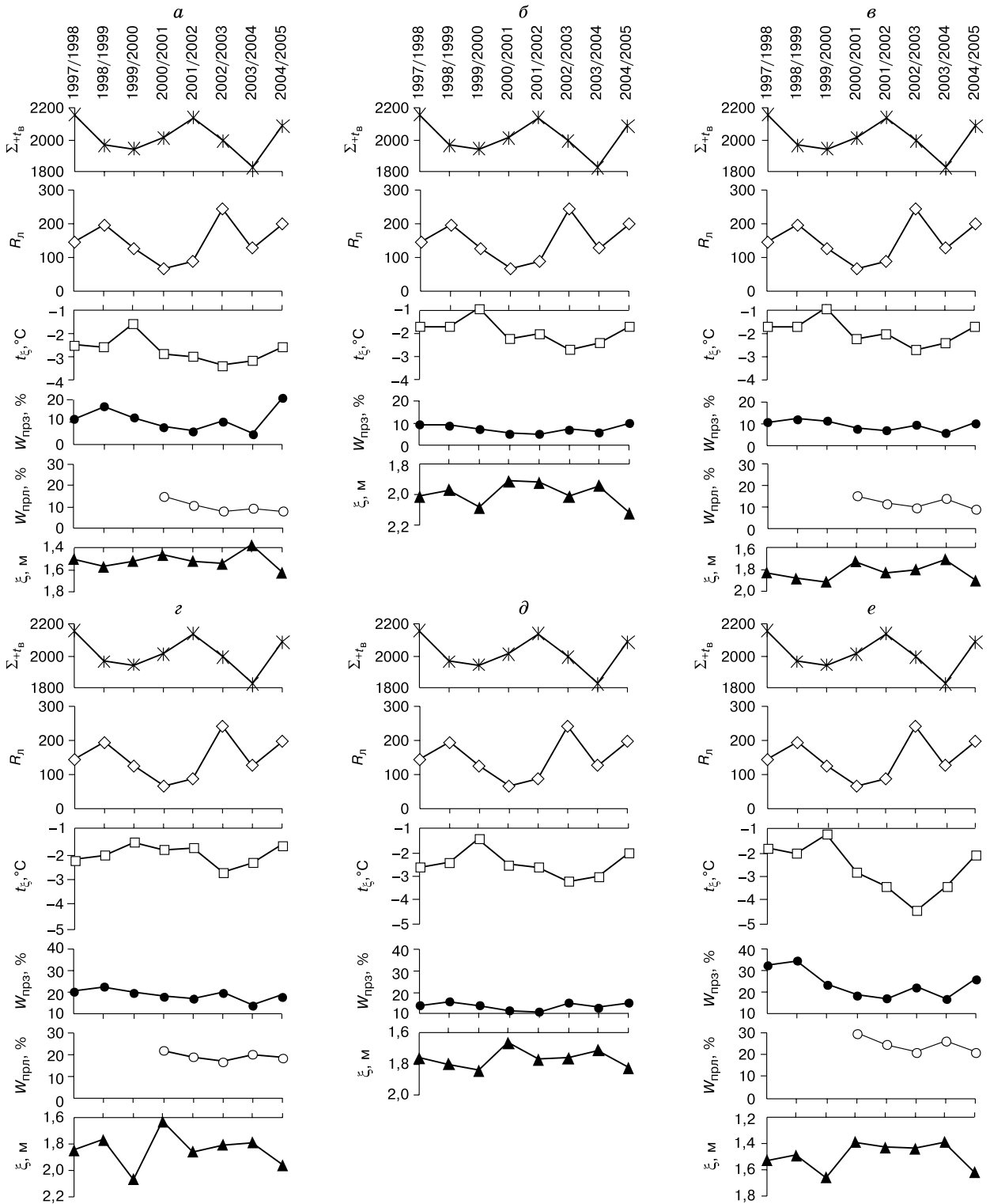
Рис. 2. Межгодовые изменения суммы положительных температур воздуха ( \Sigma_{+t_b} ), суммы осадков теплого периода ( R_n ), средней годовой температуры грунтов ( t_{\xi} ), предзимней ( W_{прз} ) и предплетней ( W_{прл} ) влажности почвогрунтов СТС (осредненные значения для всего профиля СТС) и максимальной глубины сезонного протаивания ( \xi ) на экспериментальных участках 1–6 (а–е соответственно).
